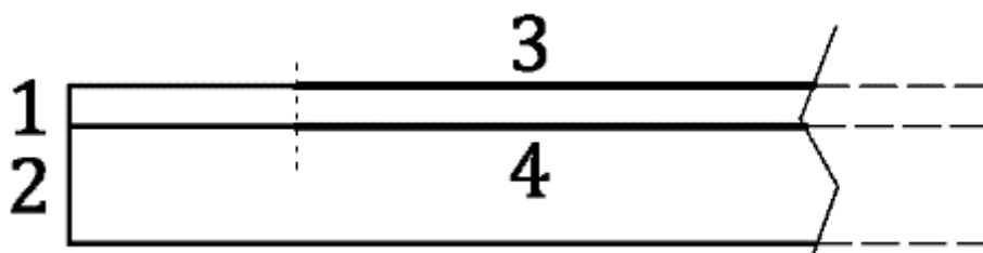
1 - фильтр; 2 – подложка, 3 – рабочая область, 4 – активная область источника Рисунок 1 — Чертеж поперечного сечения источника с фильтром
