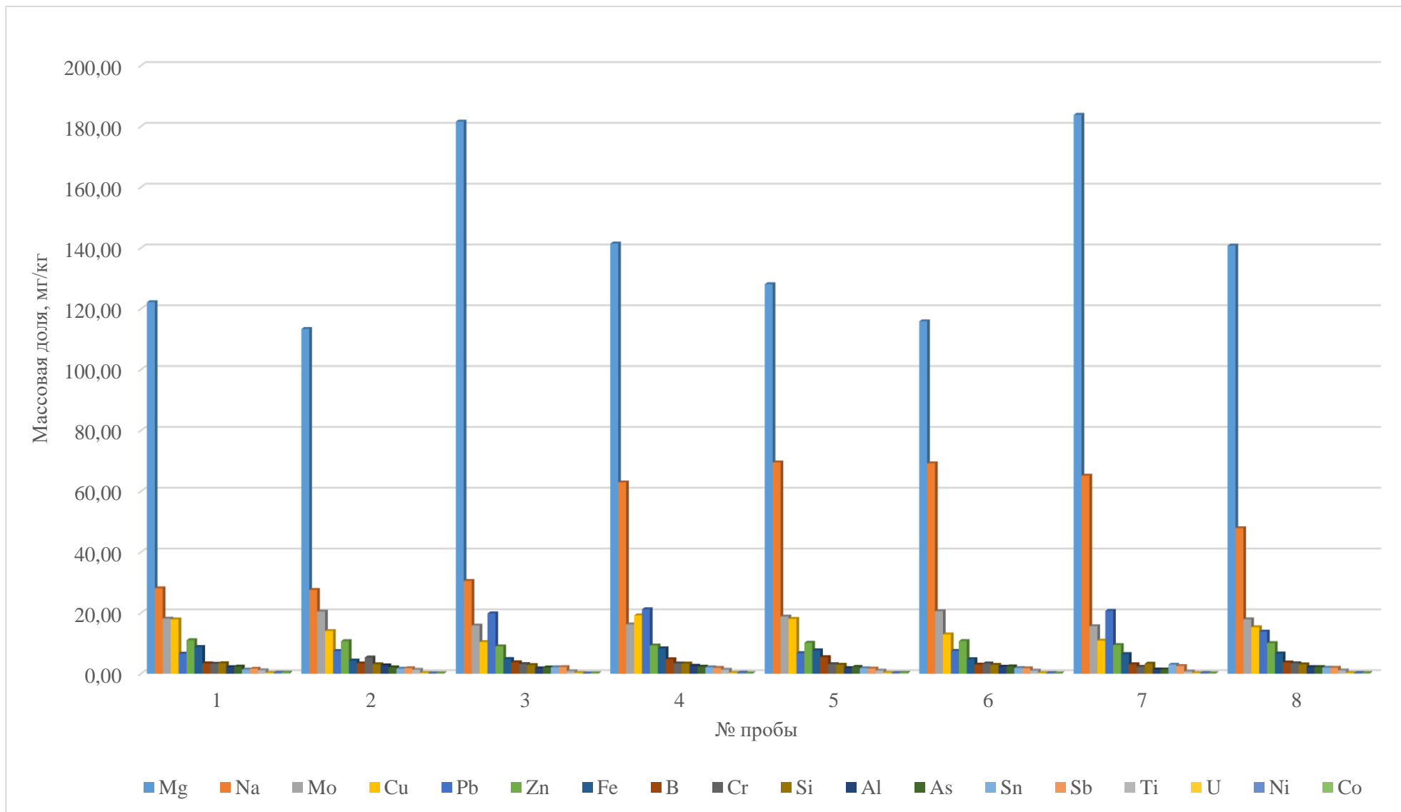
Рисунок 26 – Однородность примесного состава ЭС Мп высокой чистоты
