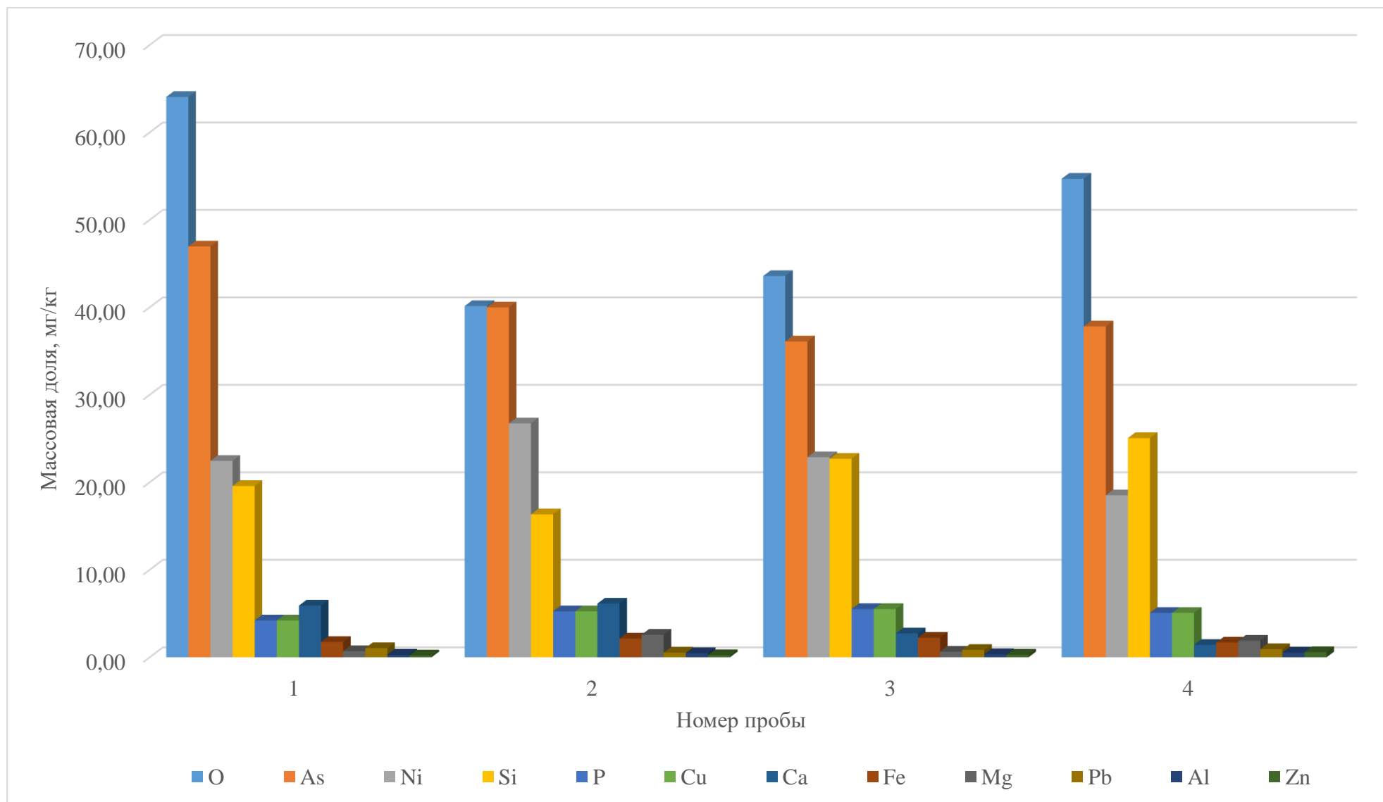
Рисунок 28 – Однородность примесного состава ЭС Со высокой чистоты
