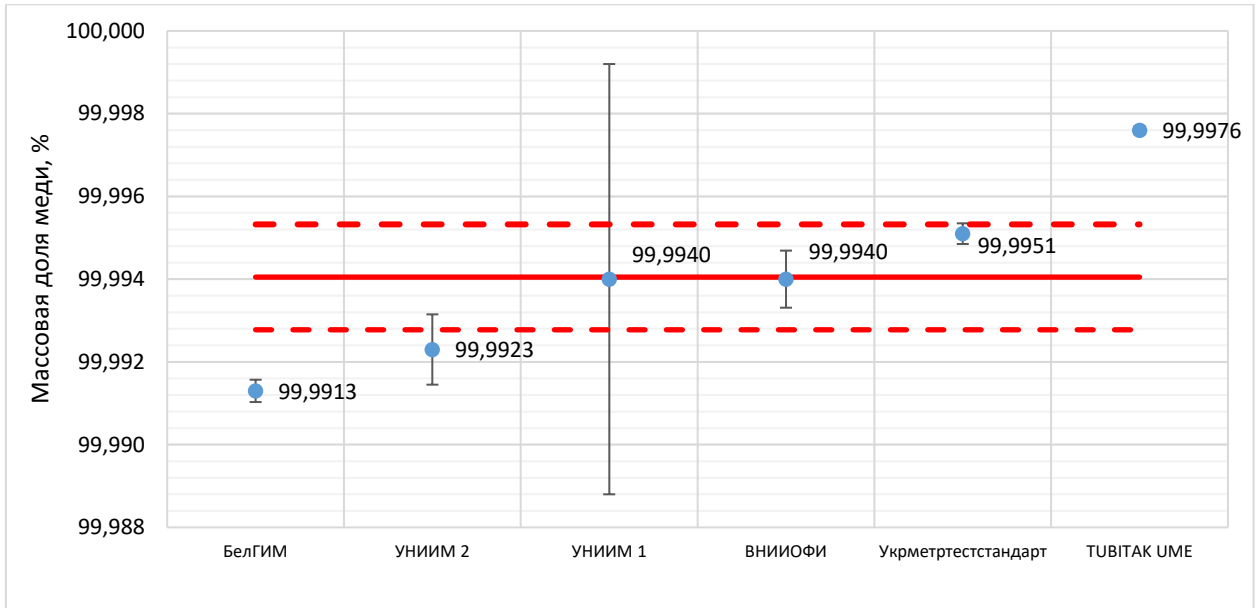
Рисунок 11 – Результаты сличений КОOMET 645/RU/14 ( k=1 ) [84]
